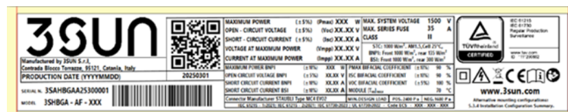
Figura 6 : esempio di etichetta di alimentazione del modulo
