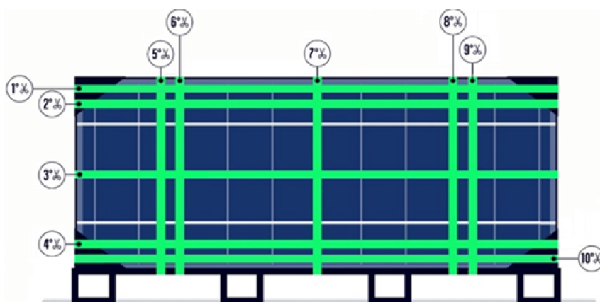
Figura 16: Posizioni delle cinghie interne.
