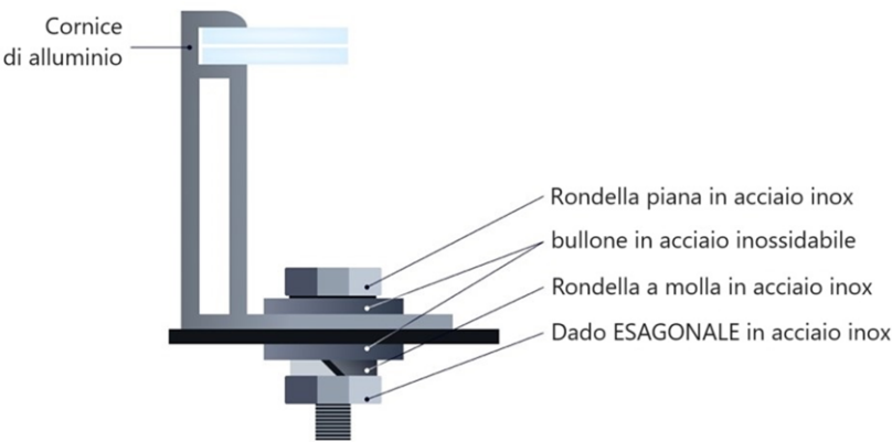
Figura 21: Modulo FV installato con metodo di montaggio a bullone.
