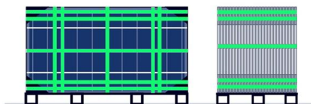
Figura 2: Scatola inferiore/superiore aperta, vista frontale e laterale
