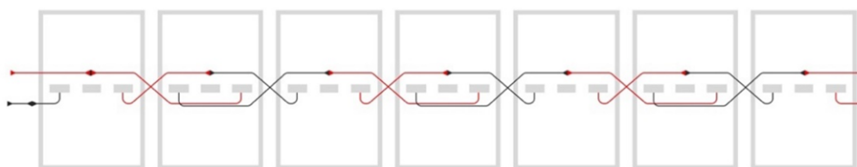
Leapfrog Wiring
