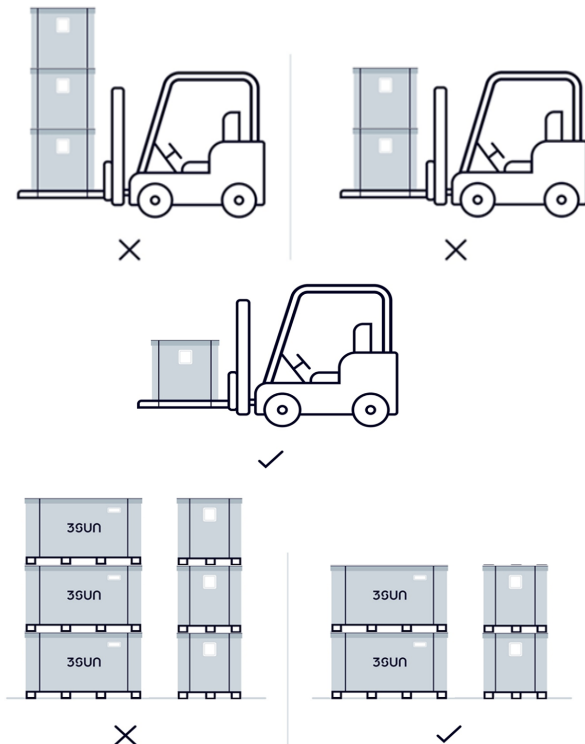
Figura 12: Non è consentito impilare oltre due scatole single
