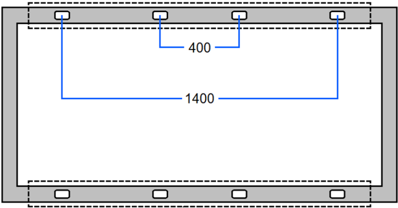
Figura 22: Posizione dei fori di montaggio della cornice.
