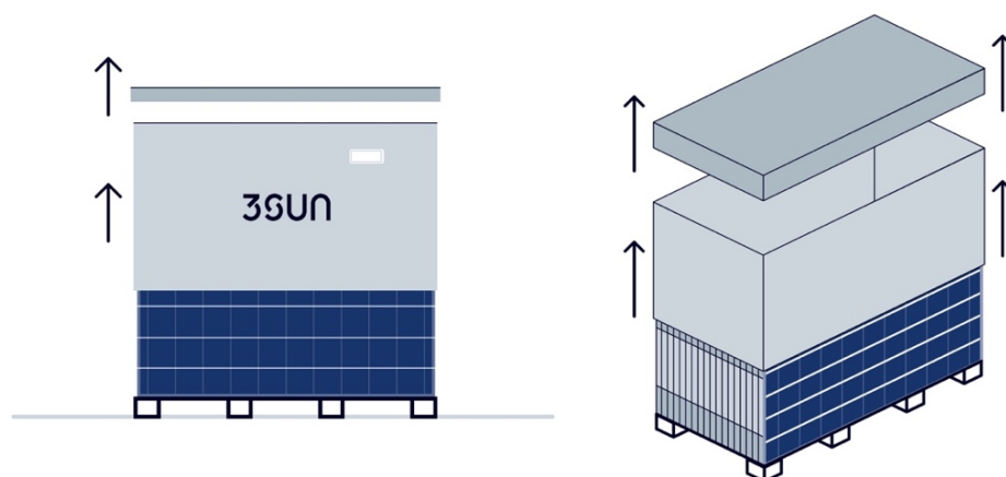
Figura 15: Rimozione del coperchio e dell'imballaggio perimetrale della scatola.
