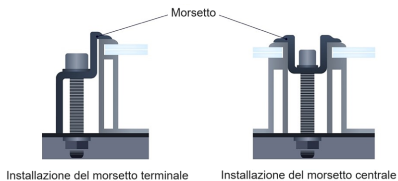
Figura 20: Esempio di installazione con morsetto.
