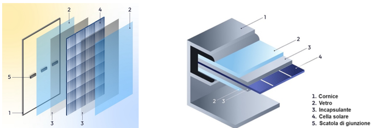
Figura 3: sezioni trasversali rappresentative dei moduli FV.
