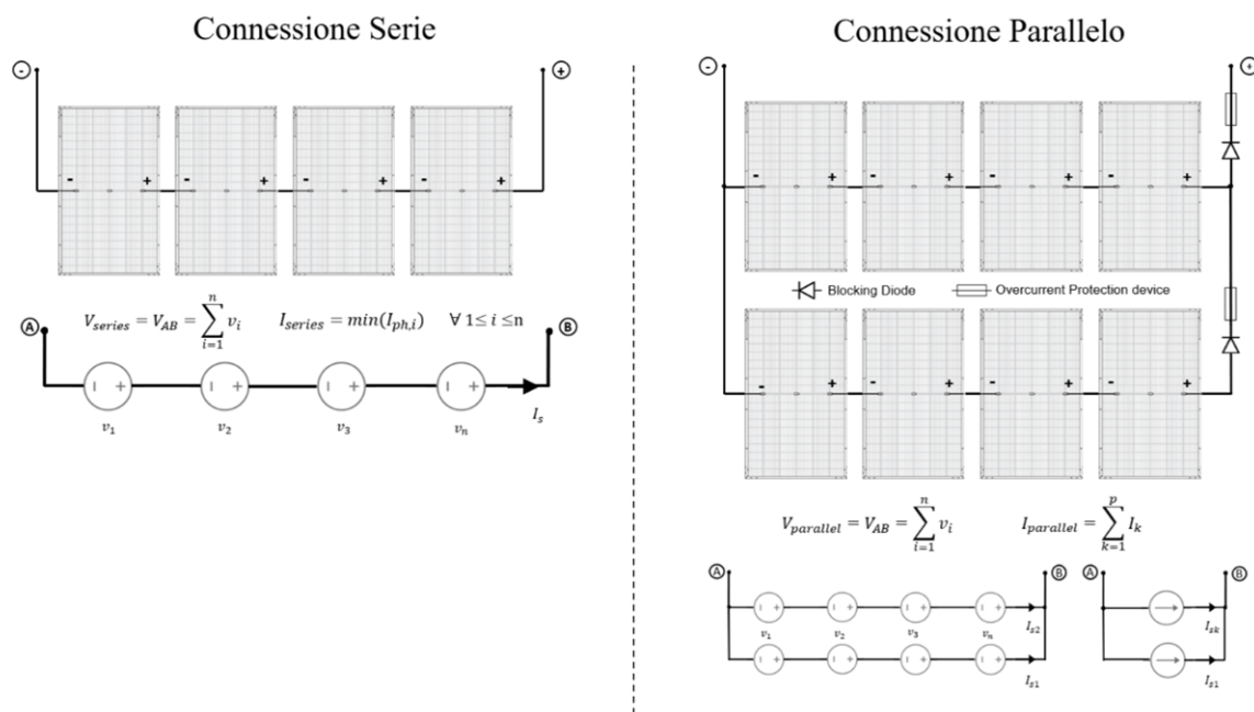
Figura 23: Schema del circuito di collegamento in serie e collegamento in parallelo
