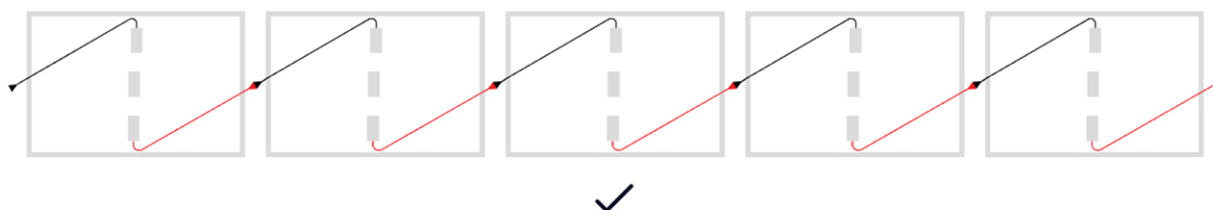
Figura 25: Daisy-Chain posizionamento e interconnessione per moduli orizzontali – in caso di cavo da 1400mm
